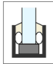
標準施工(発泡材+弾性シーラント施工)
